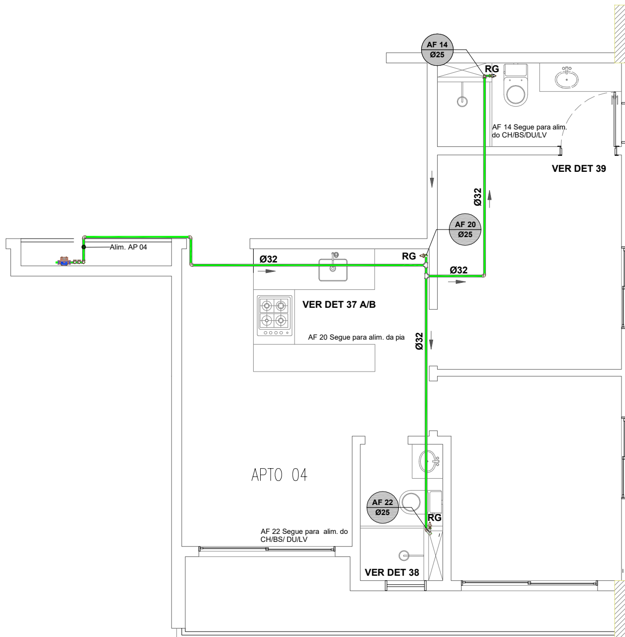
PLANTA BAIXA - APTO. 04 13° AO 14° PAVIMENTO SEM ESCALA
