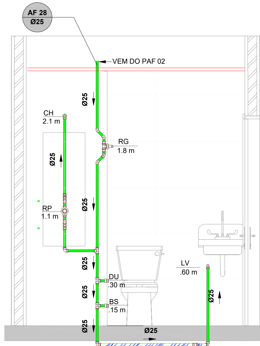
DETALHE 46
